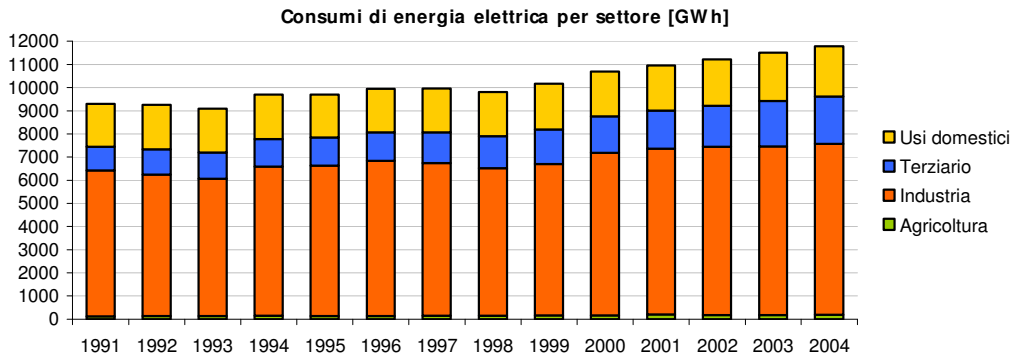
Figura 4-20: trend nei consumi di energia per settore
